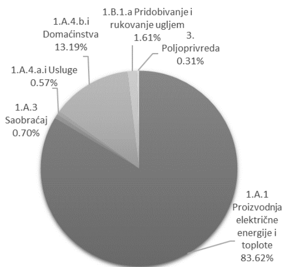
Slika 4. Emisije PM2.5 po sektorima
