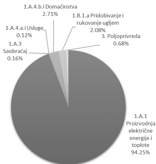
Slika 3. Emisije PM10 po sektorima
