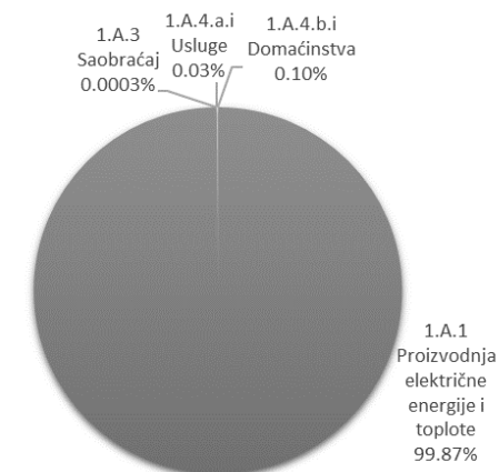
Slika 1. Emisije SOx po sektorima
