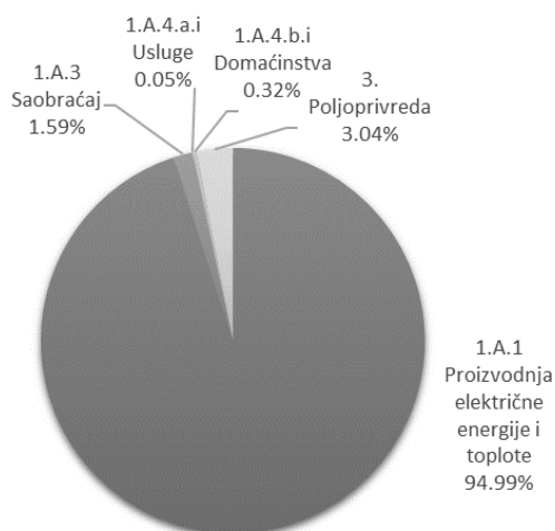
Slika 2. Emisije NOx po sektorima
